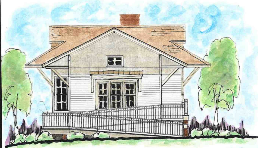
1 REAR ELEVATION A3.1 SCALE: 1/4" = 1'-0"
