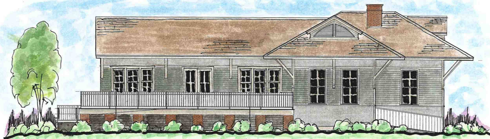
1 LEFT ELEVATION A3.2 SCALE: 1/4" = 1'-0"
