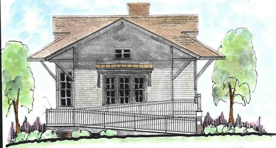
1 REAR ELEVATION A3.1 SCALE: 1/4" = 1'-0"
